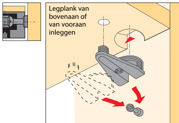
Verbindingsbeslag VB 21 voor 19 - 20 mm legplanken
